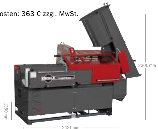
Transportstellung mit hochgeklappter Abföhrinne und eingefahrener Holzustammzuföhrung.
